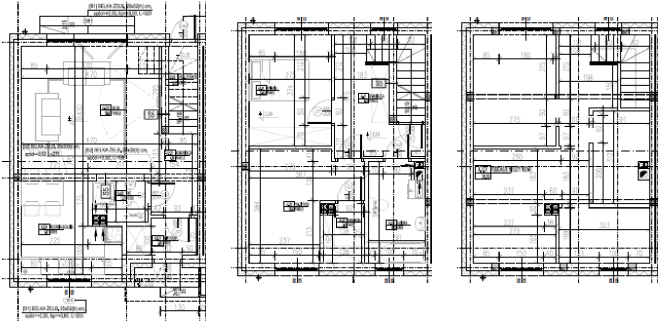
B1/1, B2/1 – parter, piętro i poddasze nieużytkowe
